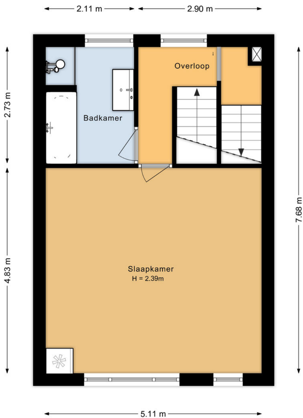
Eerste verdieping Van Panhuysstraat 62 Noordwijk
