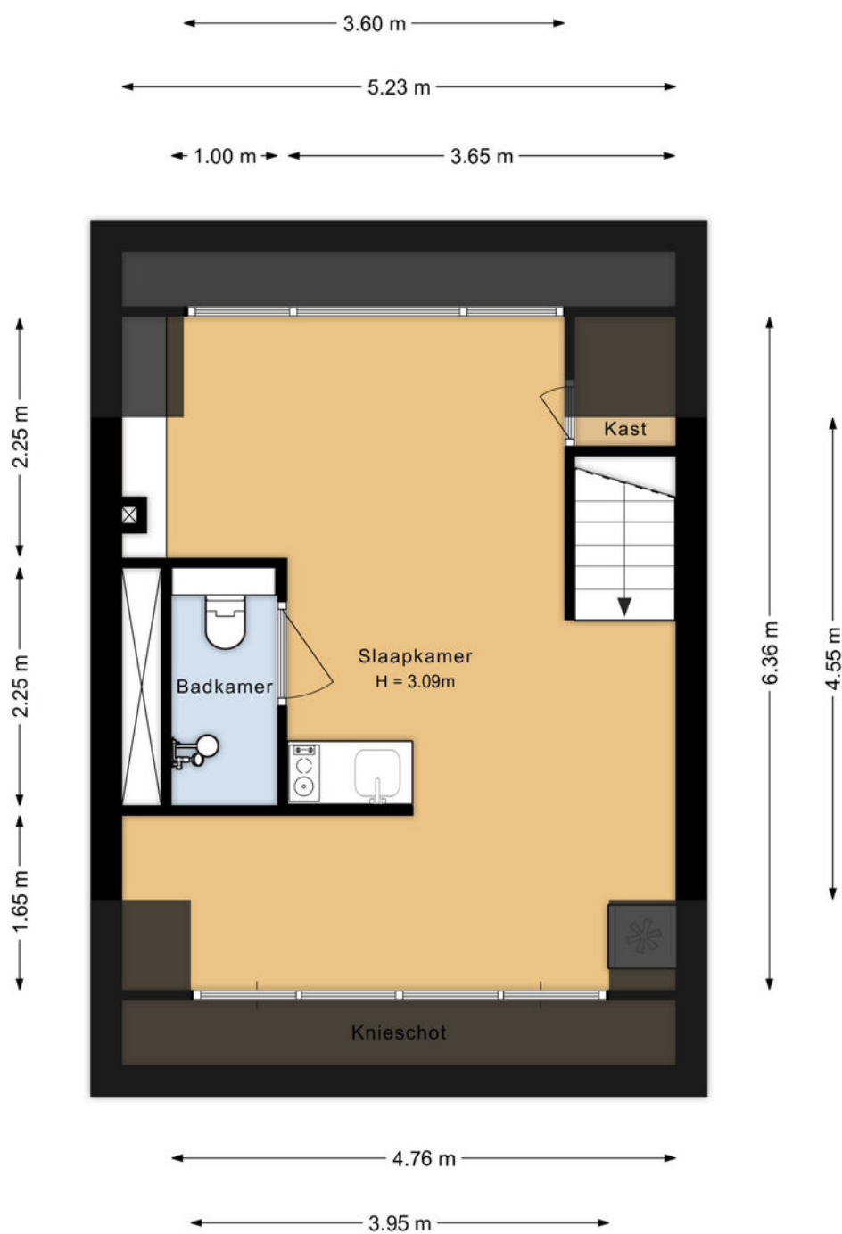
Tweede verdieping Van Panhuysstraat 62 Noordwijk
